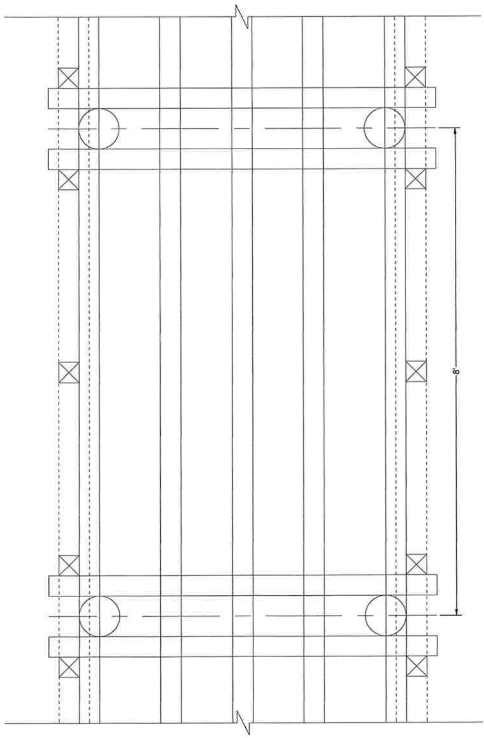
2 SECTION VIEW SCALE: 1" = 1'-0"
